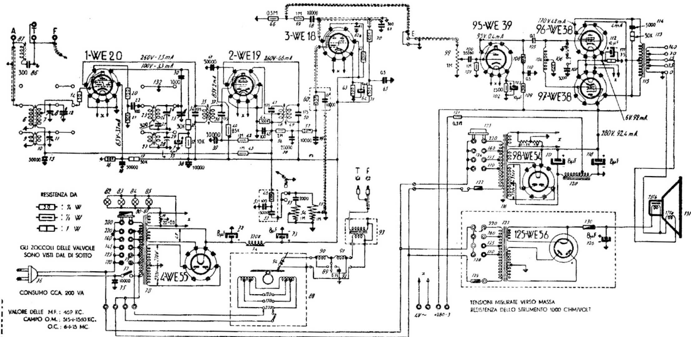
SIEMENS - Mod. 925 - Radiofonografo con due WE 38 finali in controfase. Due gamme d'onda. Media frequenza: 469 kc/s. Consumo circa 200 W. Tensioni e correnti indicate nello schema. Produzione 1945-46. (V. note taratura a parte).
